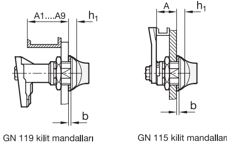
GN 119 kilit mandalları
